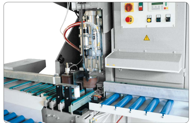
Schraubvorschubeinheit
